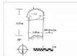
Sezione F-F' (est-ovest)
