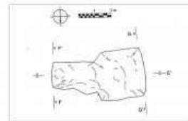
Pianta a quota 183.12 s.l.m.
