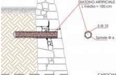
PARTICOLARE TIRANTE AD ATTRITO
