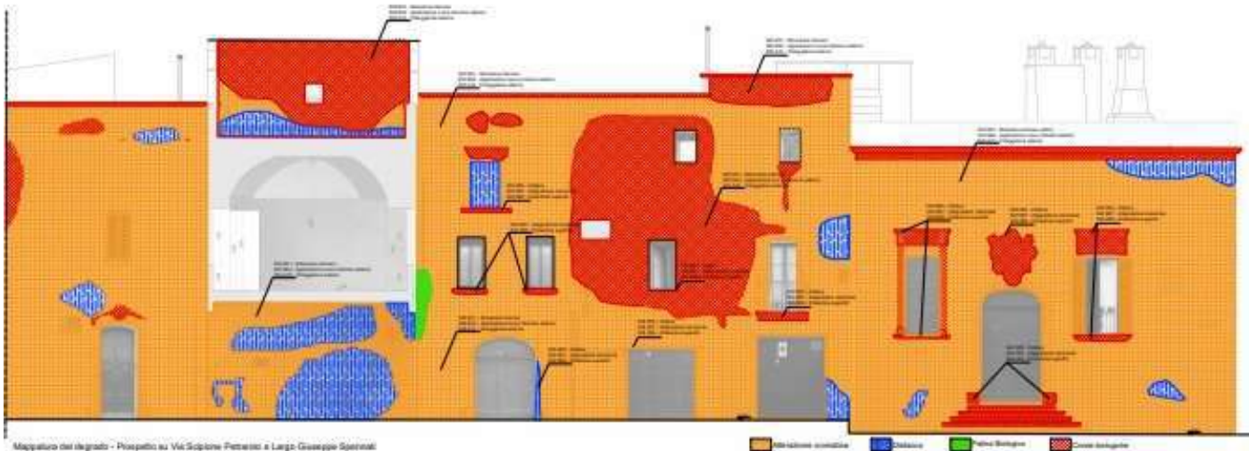
Mappatura dei degradi - Prospetto su Via Scipione Petrarco e Largo Giuseppe Spornati
