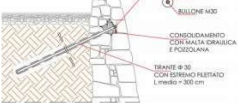
PARTICOLARE TIRANTE AD ATTRITO
